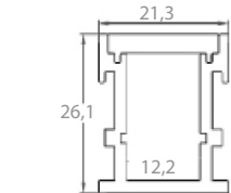
Espessura do alumínio 1,1mm
